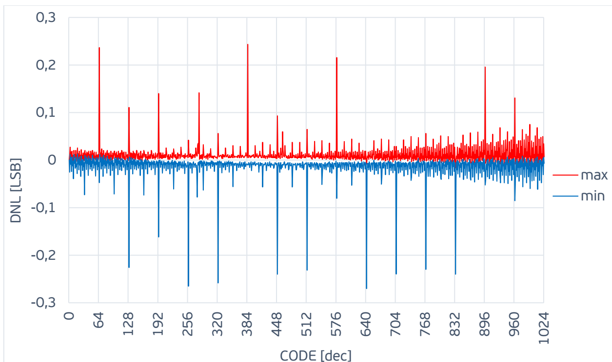
Рис. 6. Min/max DNL от входного кода при высоких температурах ( v_{dda} = v_{ddd} = v_{refp} = 1.8 \text{ В} ; T = 125^\circ\text{C} )
