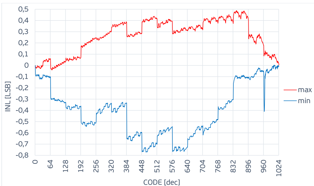
Рис. 7. Min/max INL от входного кода при низких температурах ( v_{dda} = v_{ddd} = v_{refp} = 1.8 \text{ В} ; T = -40^\circ\text{C} )
