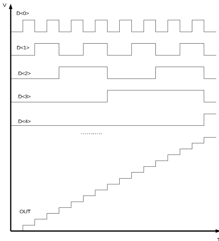
Рис. 2. Временная диаграмма TI-10DAC
