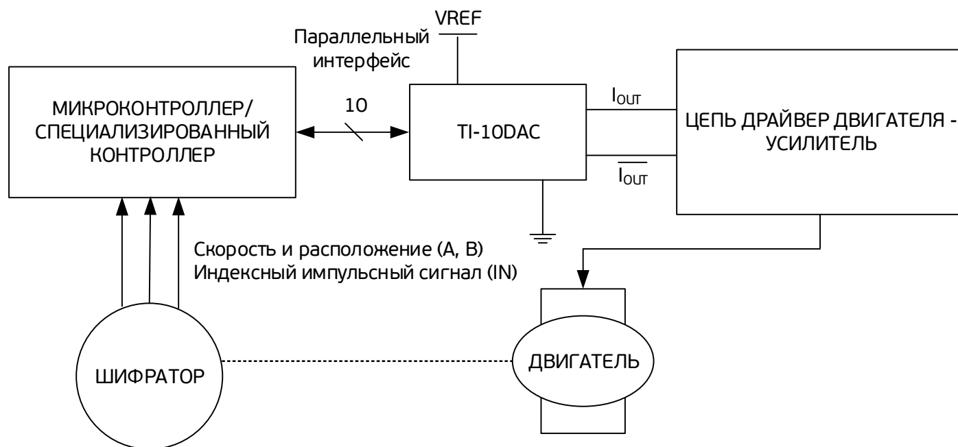
Рис. 1. Типичная схема включения TI-10DAC
