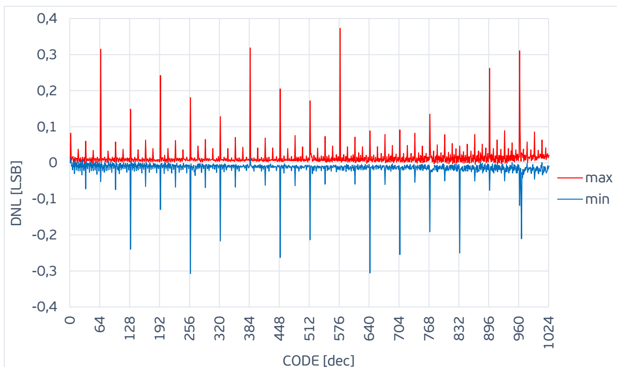
Рис. 8. Min/max DNL от входного кода при низких температурах ( v_{dda} = v_{ddd} = v_{refp} = 1.8 \text{ В} ; T = -40^\circ\text{C} )
